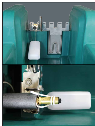
Variante I: 1x MAXIFLOW-Ventil (an Stichelung mit Frostschutz- Heizleitung 24 V, 20 W, 2 m), 1x Zusatzheizung 24 V, 180 W
