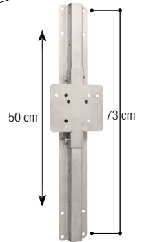
101.0433
