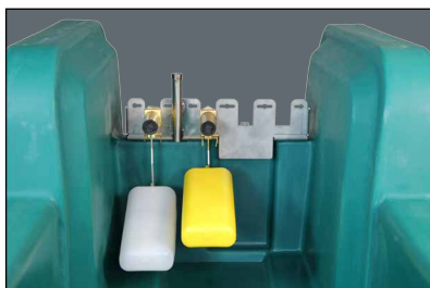
Variante D: 1x MAXIFLOW-Ventil (bis zu 40 l/min!) 1x Niederdruck-Ventil
