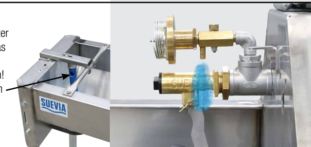
Durchlaufrohr 3/4" 131.6064
