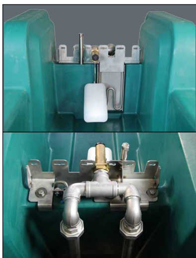
Variante G: 1x MAXIFLOW-Ventil (an Ringleitung) 1x Zusatzheizung 24 V, 180 W
