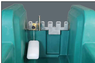
Variante A: 1x MAXIFLOW-Ventil (bis zu 40 l/min!) Auslieferungszustand Mod. 6523
