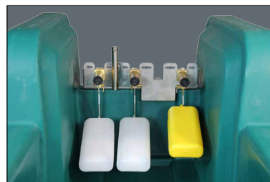
Variante F: 2x MAXIFLOW-Ventil (bis zu 80 l/min!) 1x Niederdruck-Ventil
