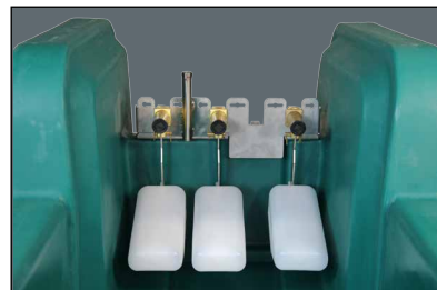
Variante C: 3x MAXIFLOW-Ventil (bis zu 120 l/min!)
