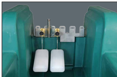
Variante B: 2x MAXIFLOW-Ventil (bis zu 80 l/min!)
