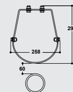
100.1239 + Zubehör für Ringleitung und Zusatzheizung
